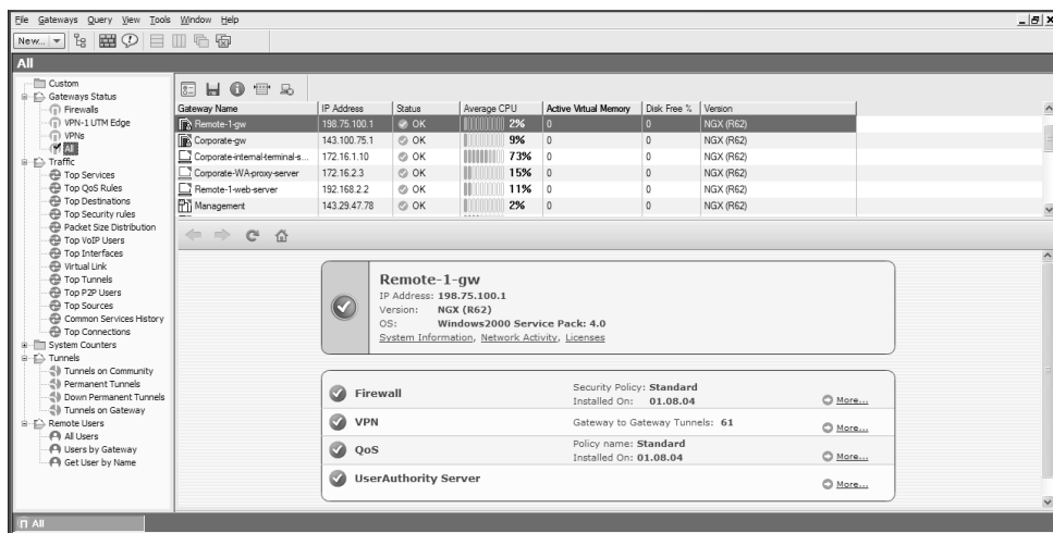
Abbildung 5.9: SmartView Monitor
