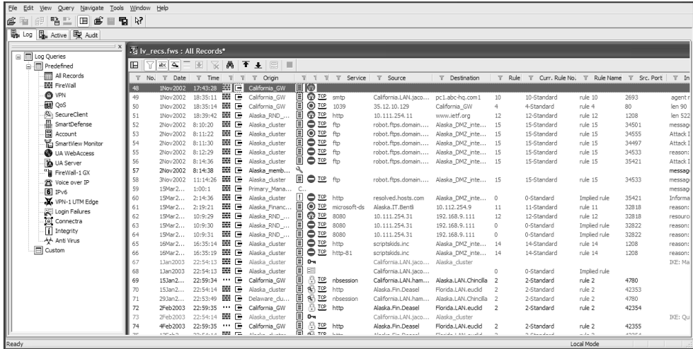
Abbildung 5.8: SmartView Tracker
