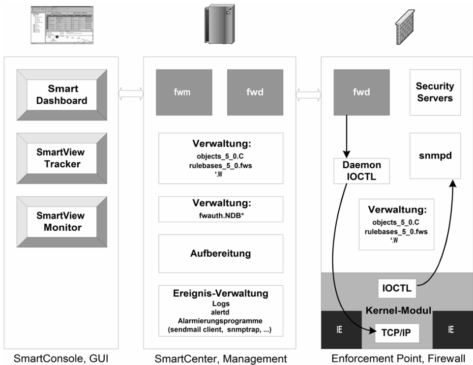
Abbildung 5.2: Zusammenhang der einzelnen Komponenten von NGX
