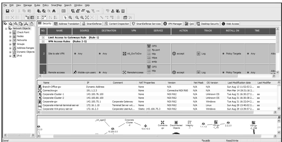
Abbildung 5.7: SmartDashboard
